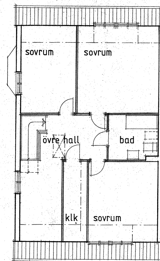
ÖVERPLAN
