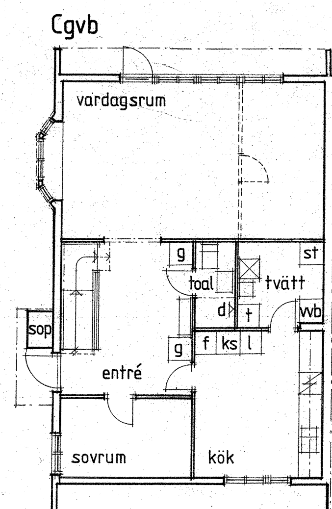
ENTRÉPLAN
