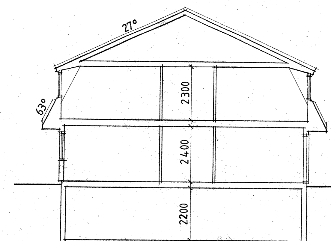
SEKTION
