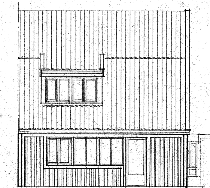
TRÄDGÅRDSFASAD Cgvb
