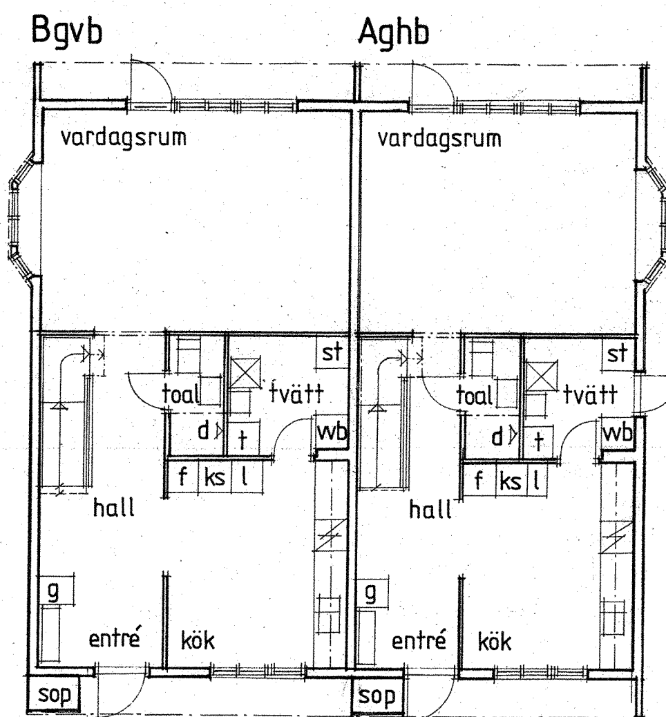
ENTRÉPLAN
