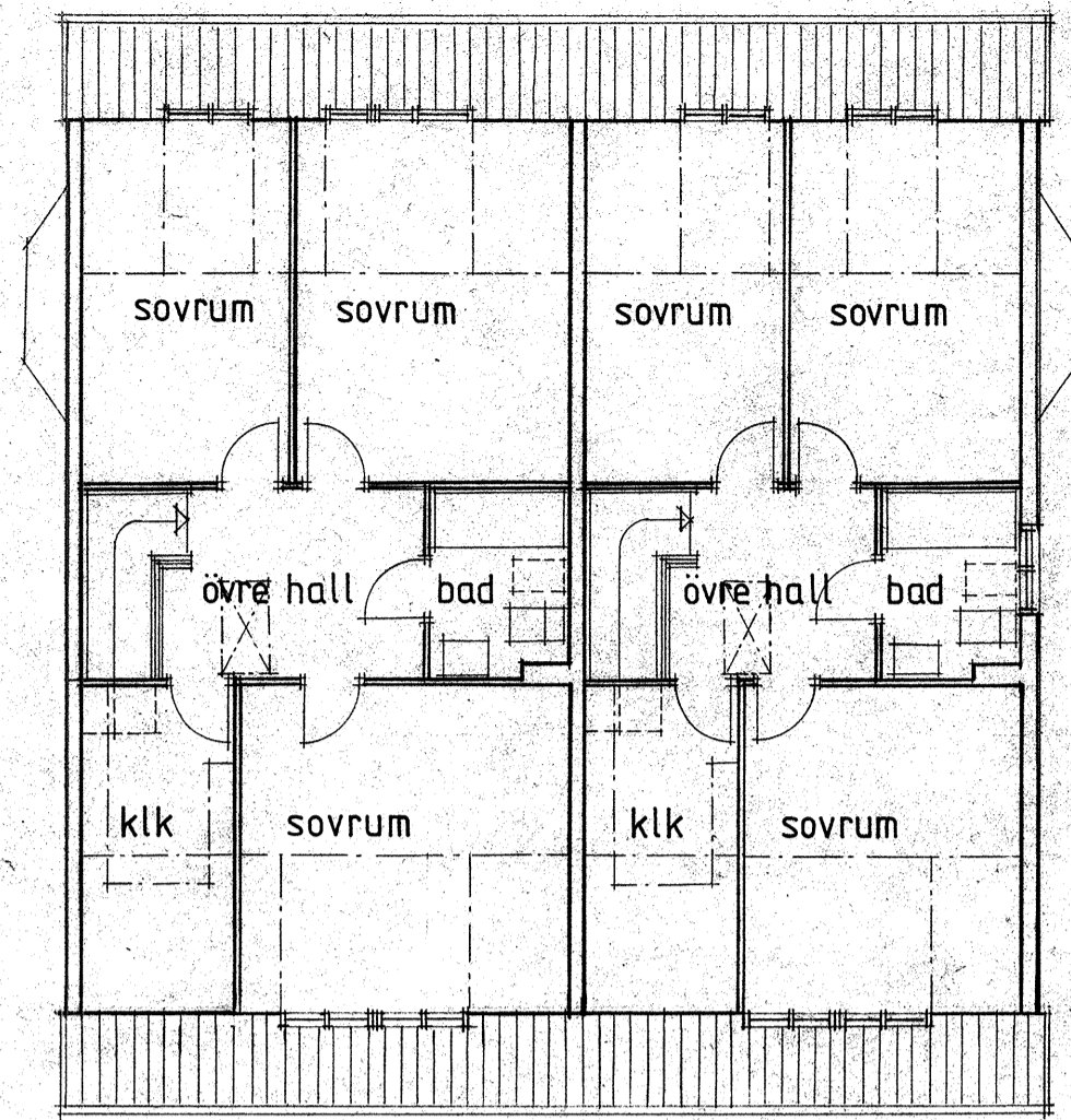
ÖVERPLAN
