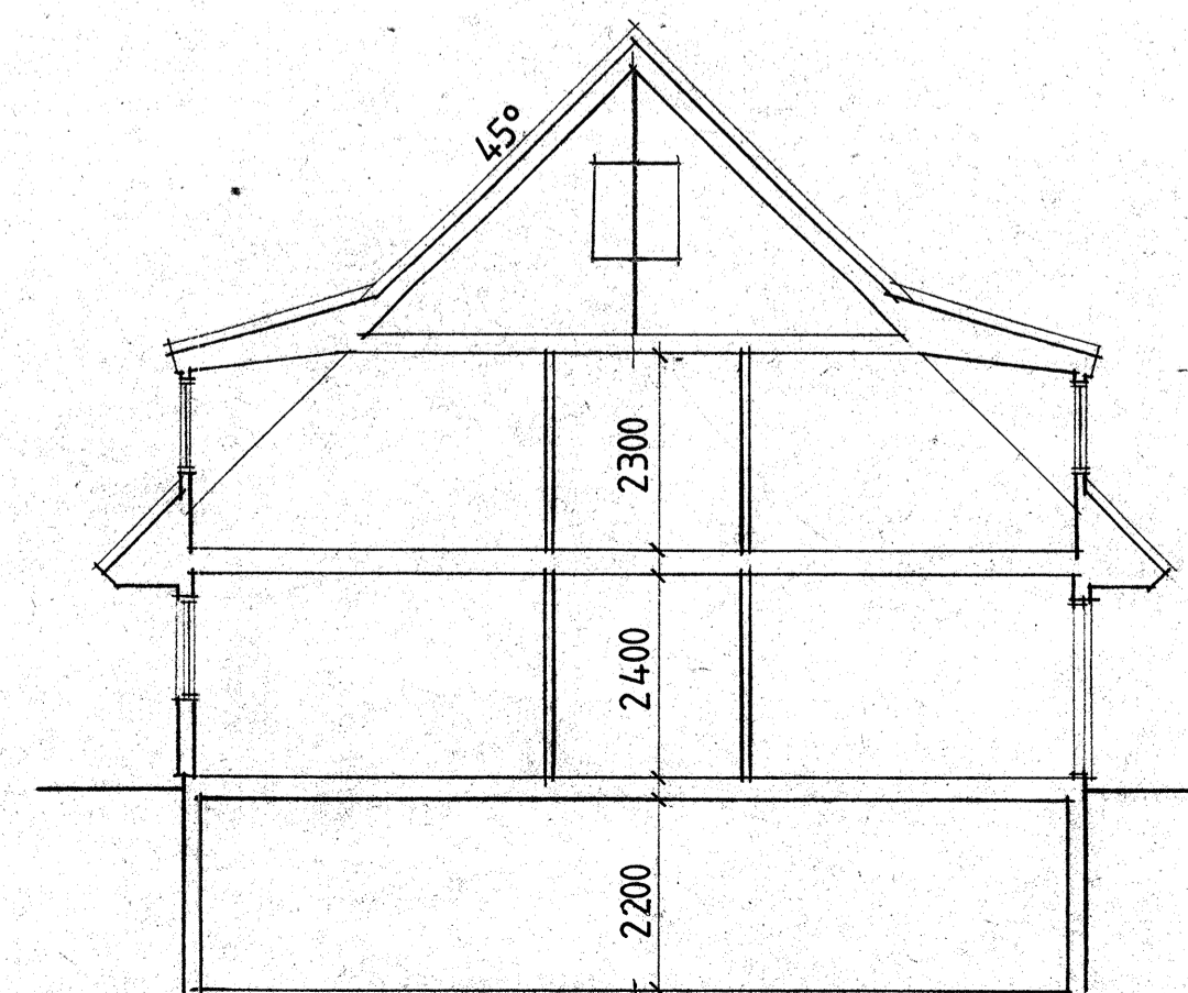
SEKTION
