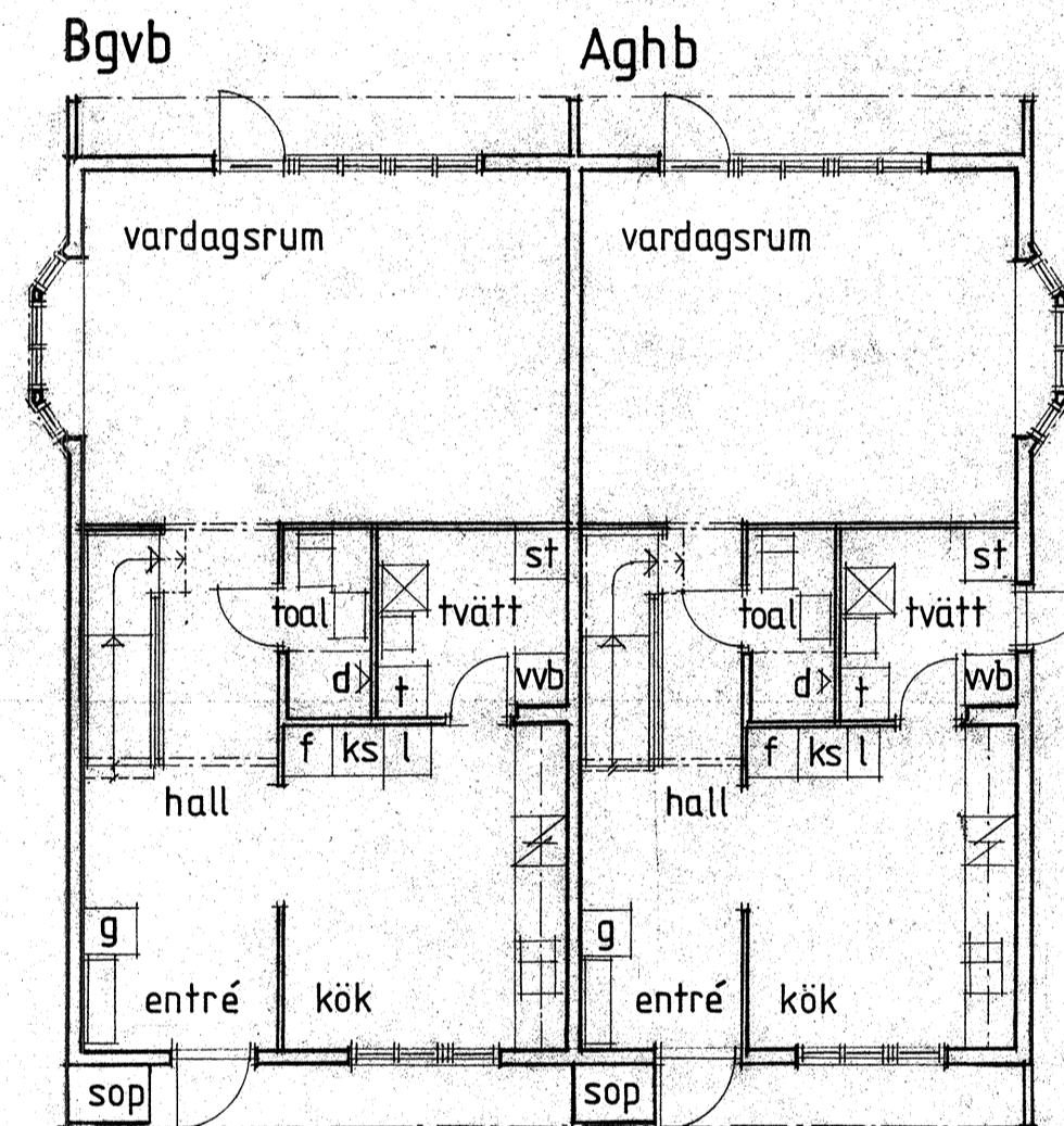
ENTRÉPLAN
