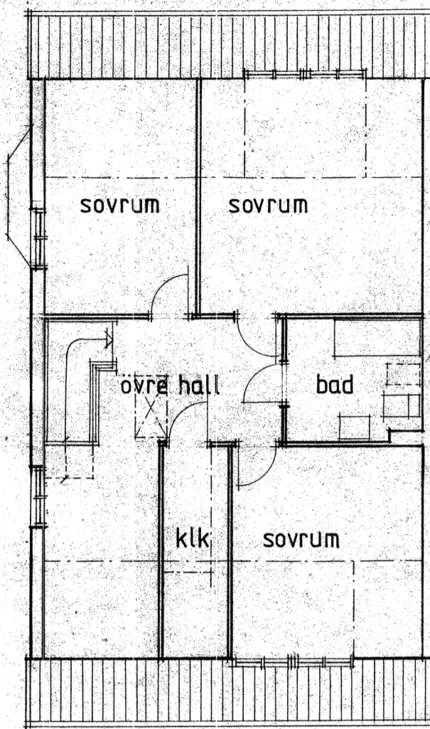
ÖVERPLAN
