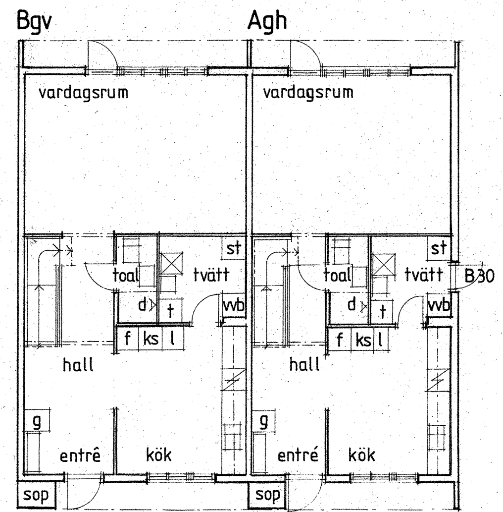
ENTRÉPLAN
