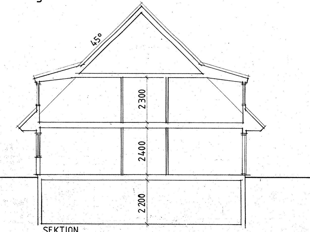
SEKTION
