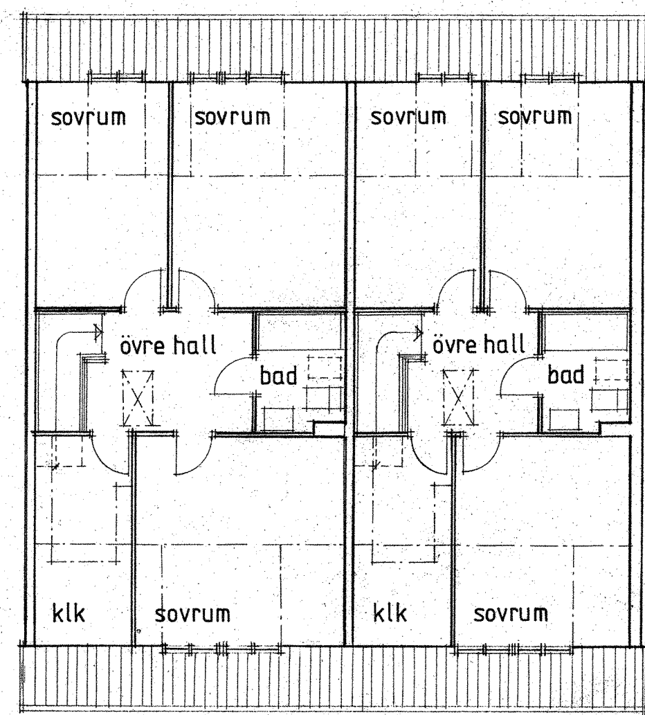
ÖVERPLAN
