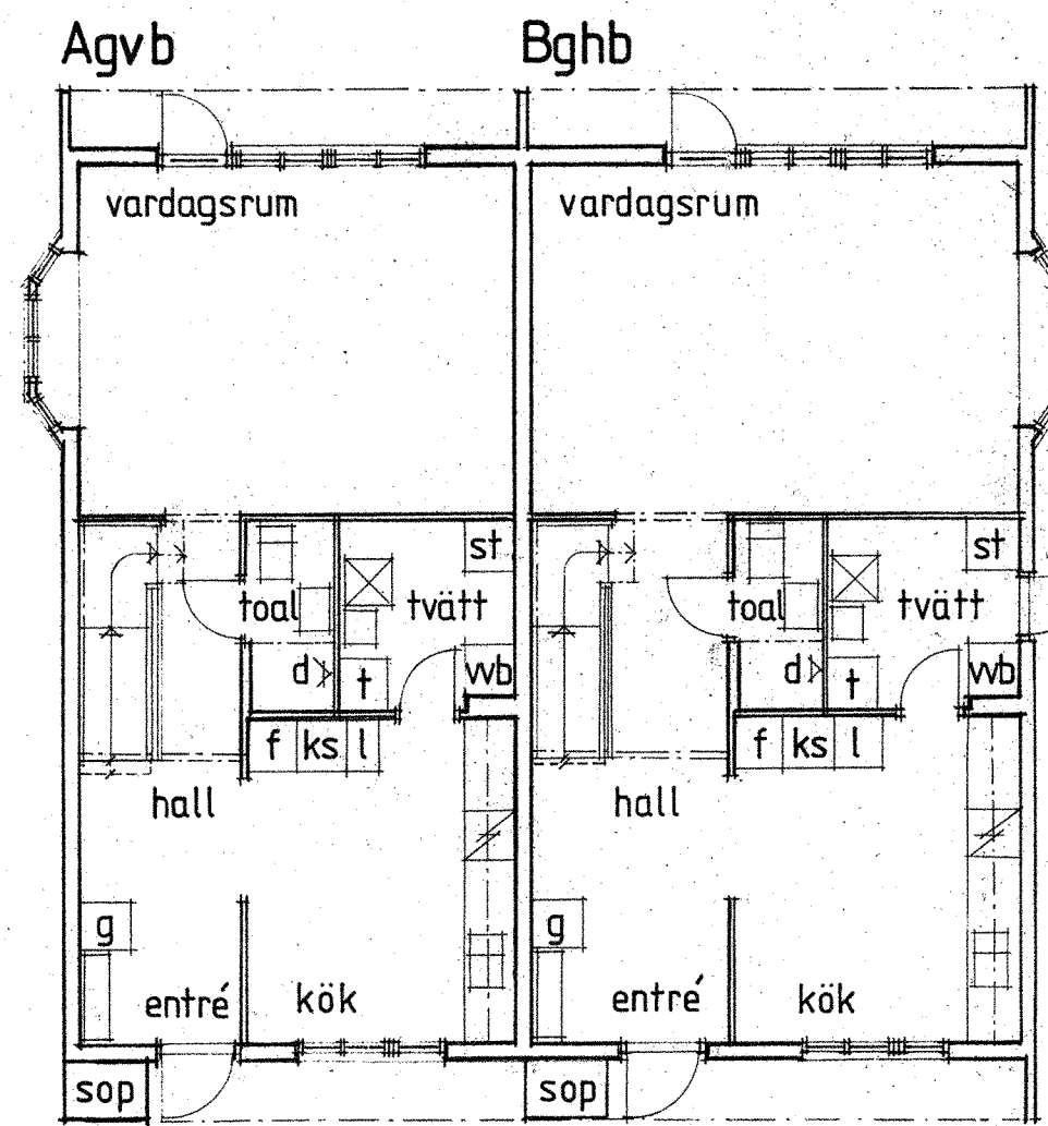
ENTRÉPLAN
