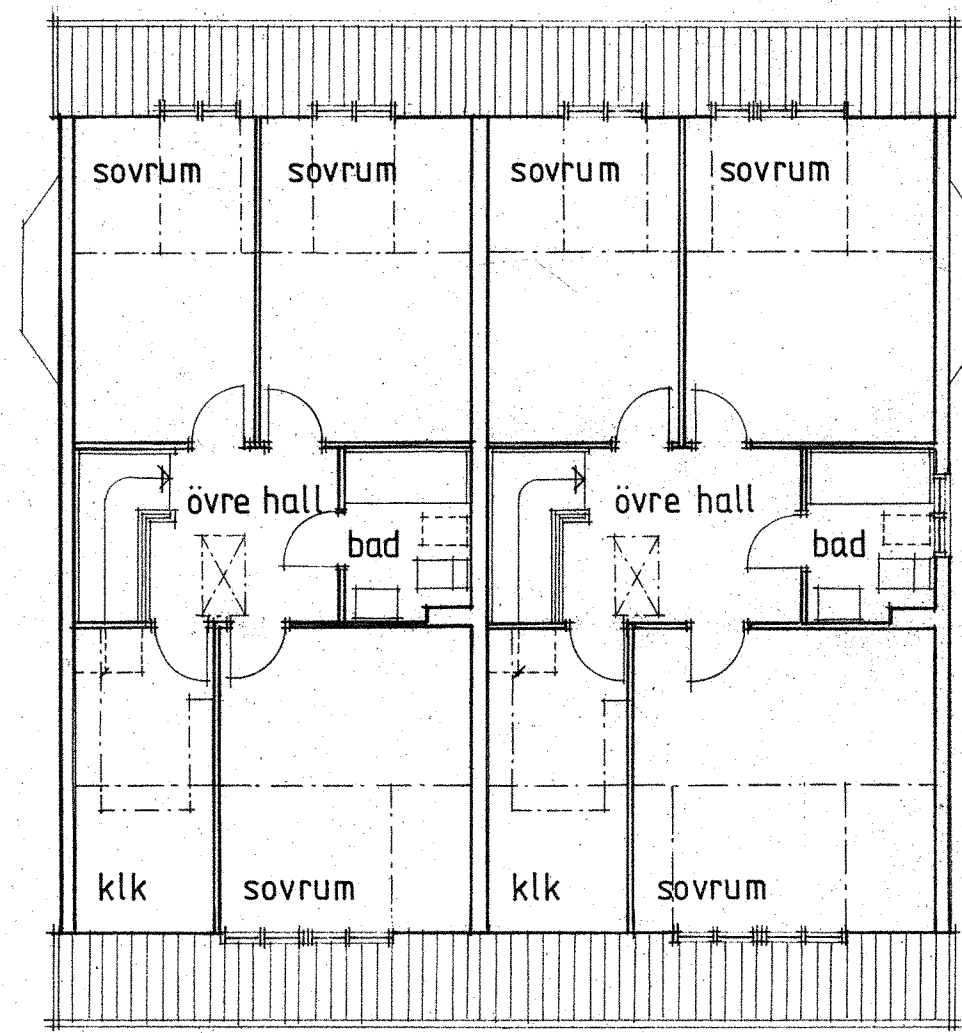
ÖVERPLAN
